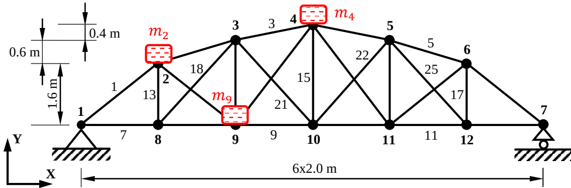
Şekil 1. Kafes köprü modelinin geometrisi
